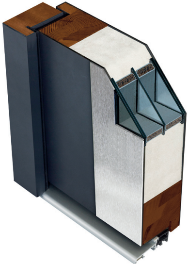
PRZEKRÓJ SKRZYDŁA Z OŚCIEŻNICĄ ENERGO
