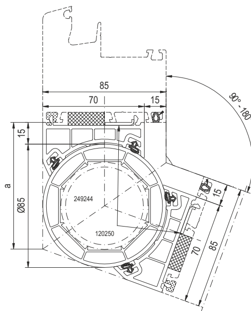
POŁOŻENIE RURY
