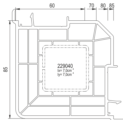
łącznik kątowy 90° Aluplast
