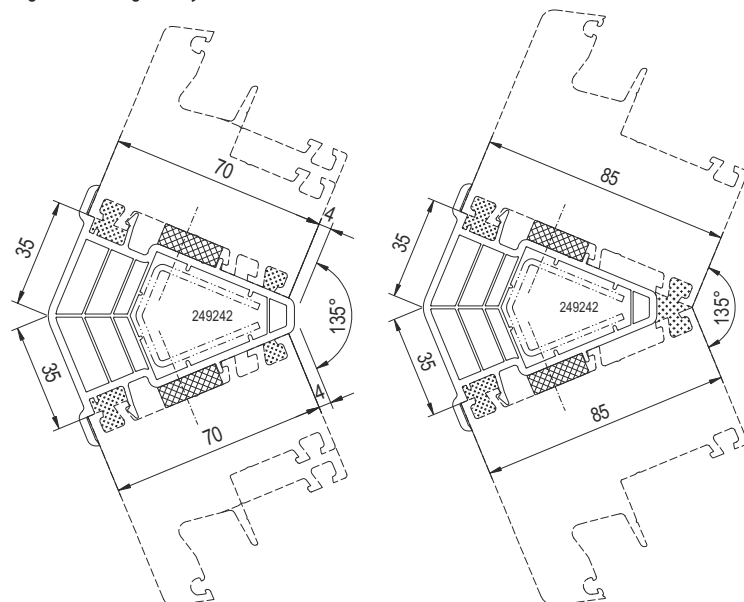
łącznik kątowy 135° Aluplast
