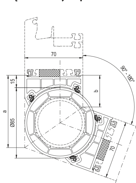
łącznik rurowy Aluplast
