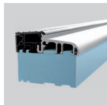
ABDICHTUNG UNTER DER SCHWELLE 60 x 30 x 1100mm
