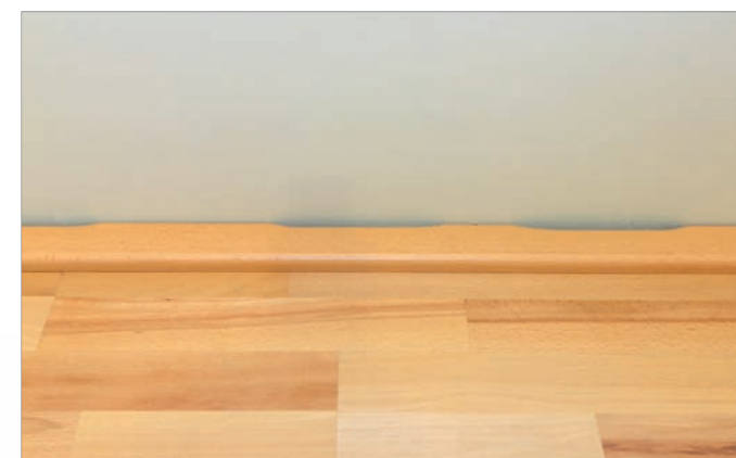
Zdjęcie 24. Przy ścianach i słupach musimy zostawić szczelinę dylatacyjną o szerokości około 15 mm. Szczelina ta pozwoli na swobodną zmianę wymiarów deski pod wpływem zmian ciepłno-wilgotnościowych. Po ułożeniu całej powierzchni podłogi montujemy listwy przyściennie ze szczeliną wentylacyjną.
